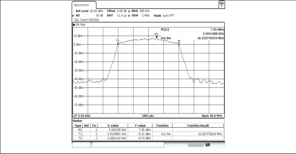
11A-Ant1-5260
