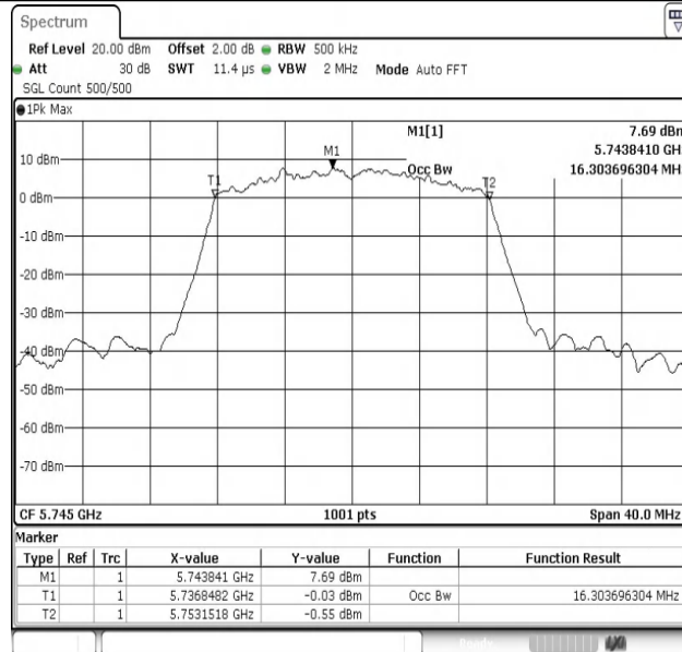
11A-Ant1-5745
