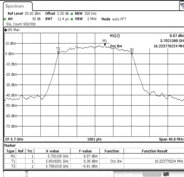
11A-Ant1-5700
