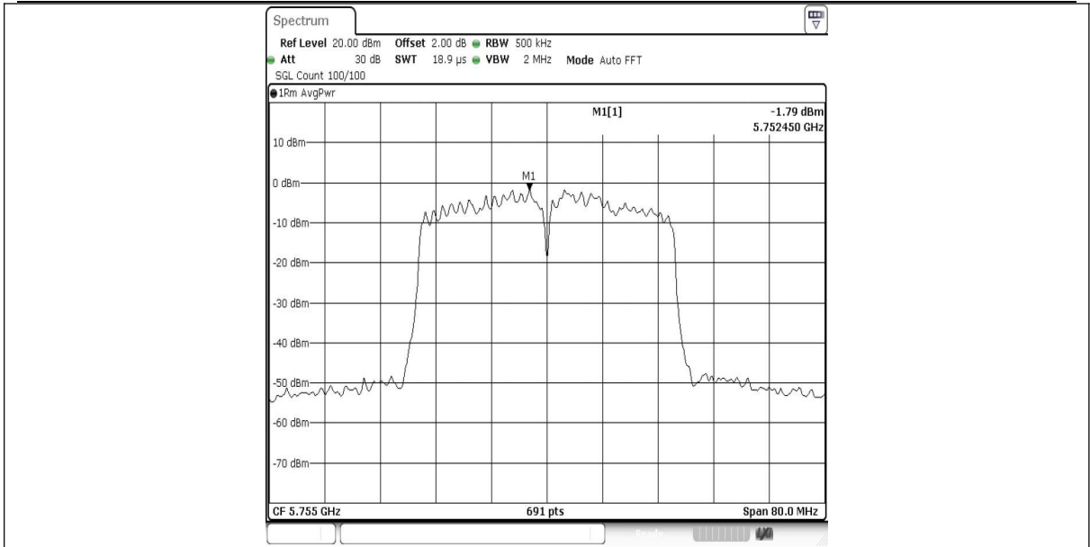
11N40SISO-Ant1-5755-PASS
