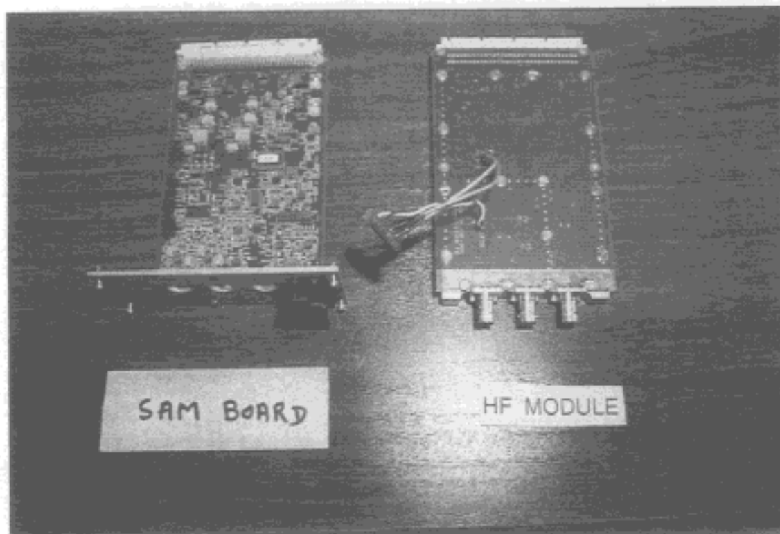
8-15 SAM component side module ( SAM BF 2480 and HF 2439 module )
