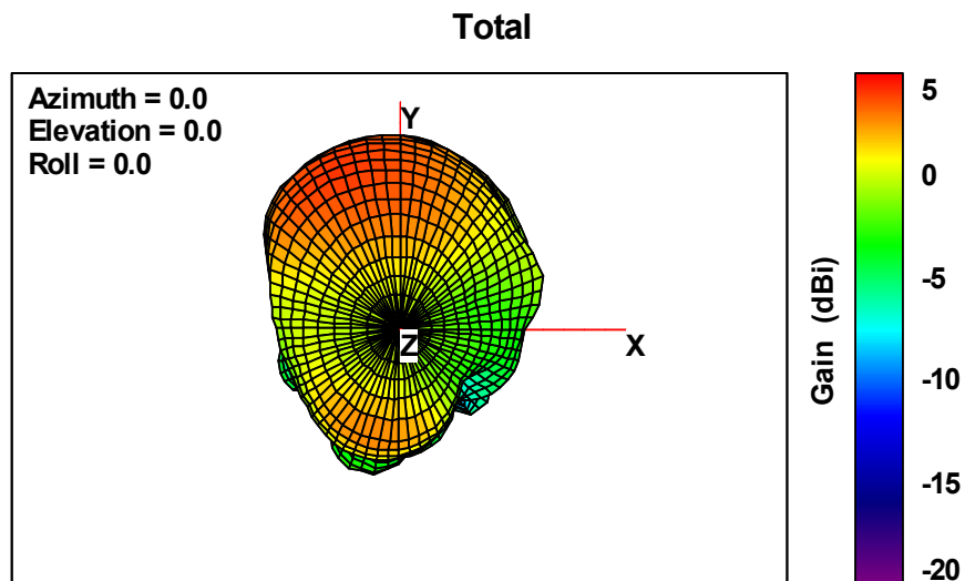
2.4GHz Ant0
