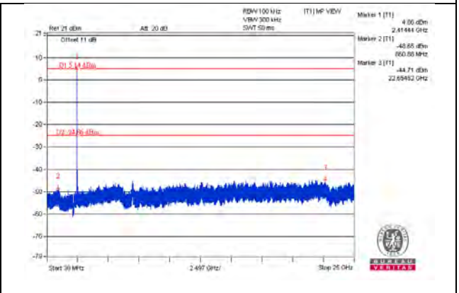
CH 6
