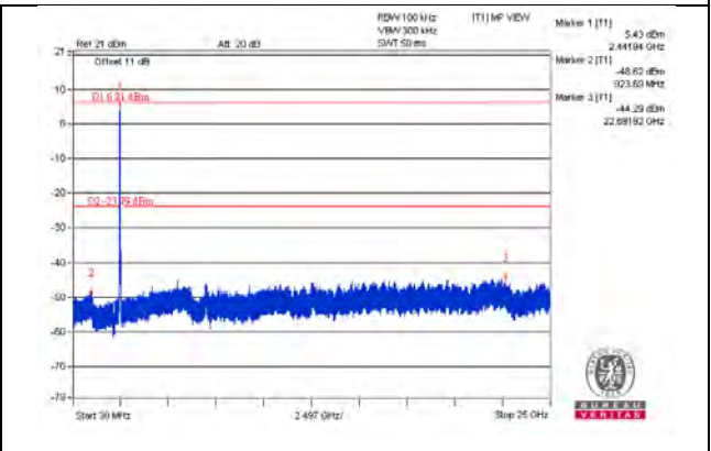
CH 9
