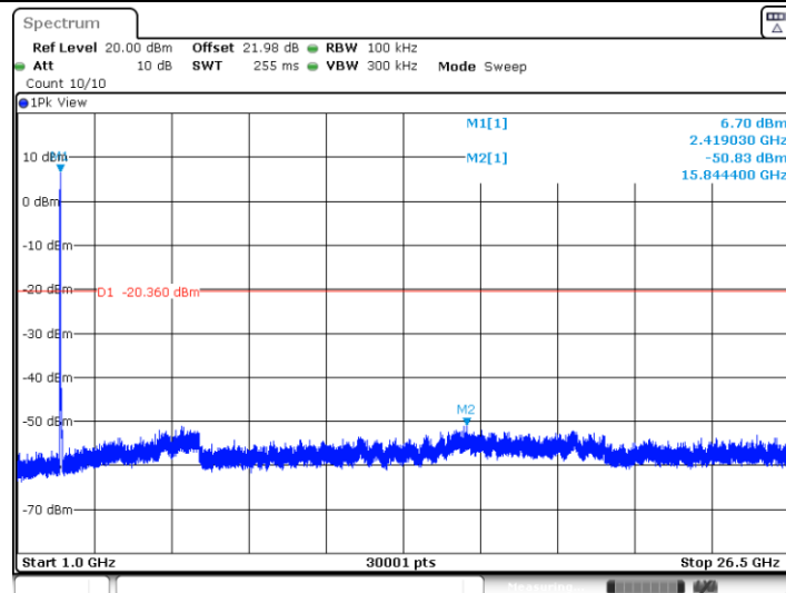
11BE20MIMO_Ant4_2412_1000~26500
