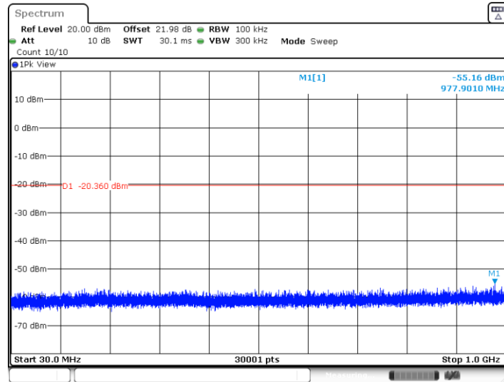
11BE20MIMO_Ant4_2412_30~1000
