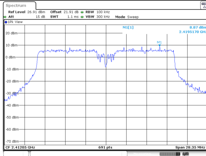
11AX20MIMO_Ant1_2412_52Tone_RU4
