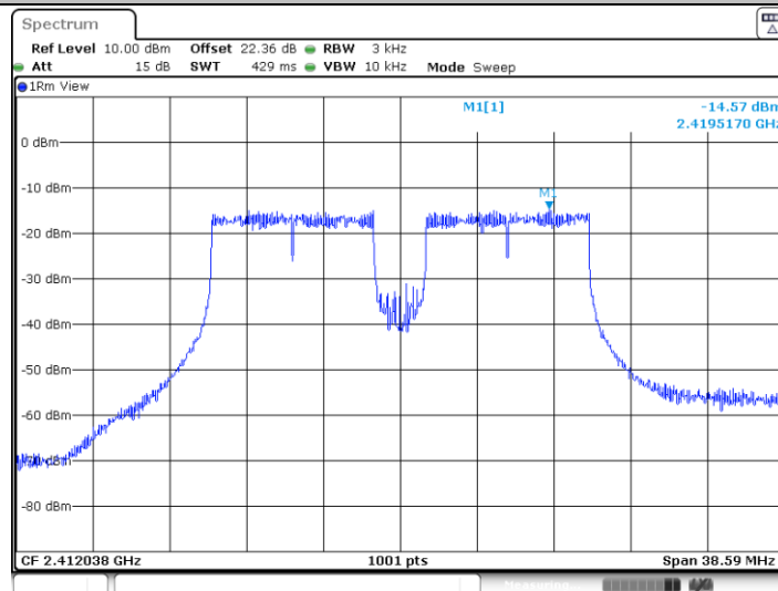
11AX20MIMO_Ant2_2412_52Tone_RU4
