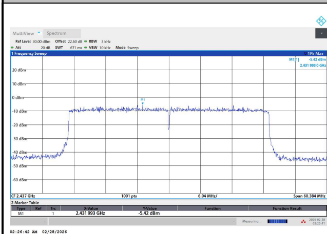
MIMO Ant. 3
