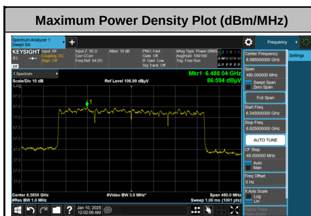
<802.11be EHT320>
