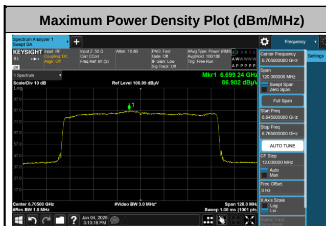
<802.11be EHT80>
