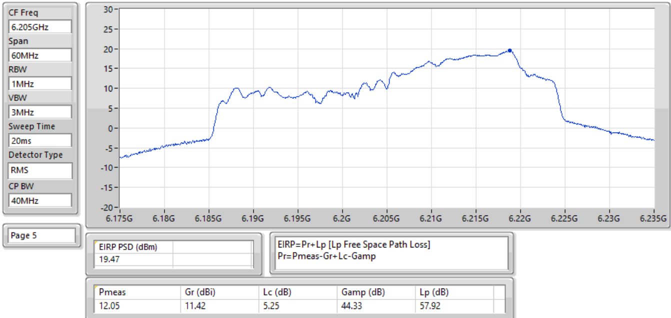
EIRP PSD;Band:6.2G;be40,BF;BWch:40MHz;Nss:1,(M0);Nant:4;Ch:6205MHz;TX
