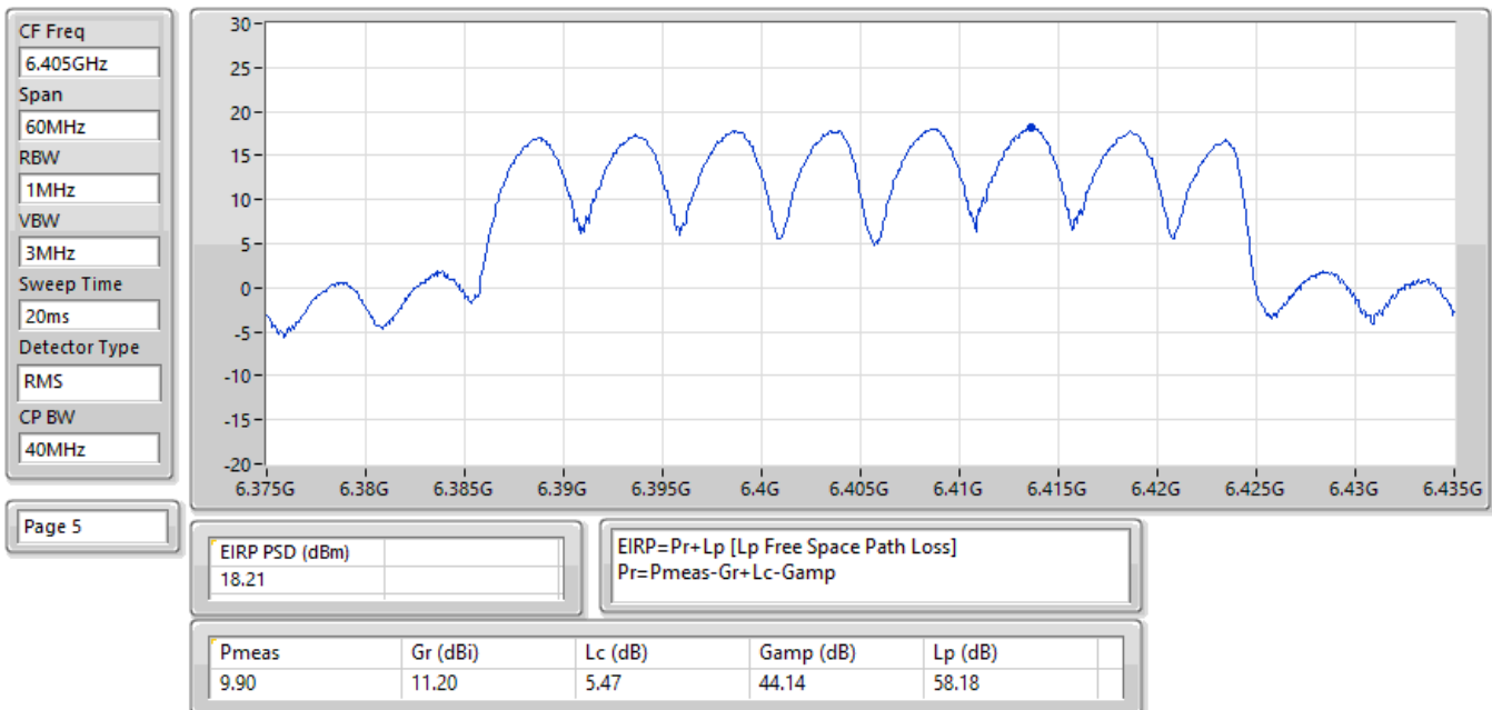
EIRP PSD;Band:6.2G;be40;BWch:40MHz;Nss:1,(M0);Nant:4;Ch:6405MHz;TX
