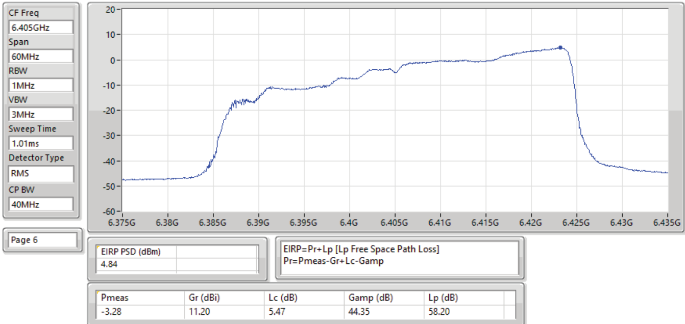
EIRP PSD;Band:6.2G;be40,BF;BWch:40MHz;Nss:1,(M0);Nant:4;Ch:6405MHz;TX
