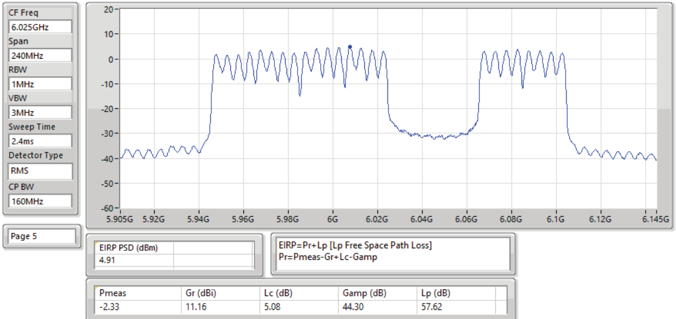
EIRP PSD;Band:6.2G;be160;BWch:160MHz;Nss:1,(M0),RU996+RU484 MRU 3;Nant:4;Ch:6025MHz;TX
