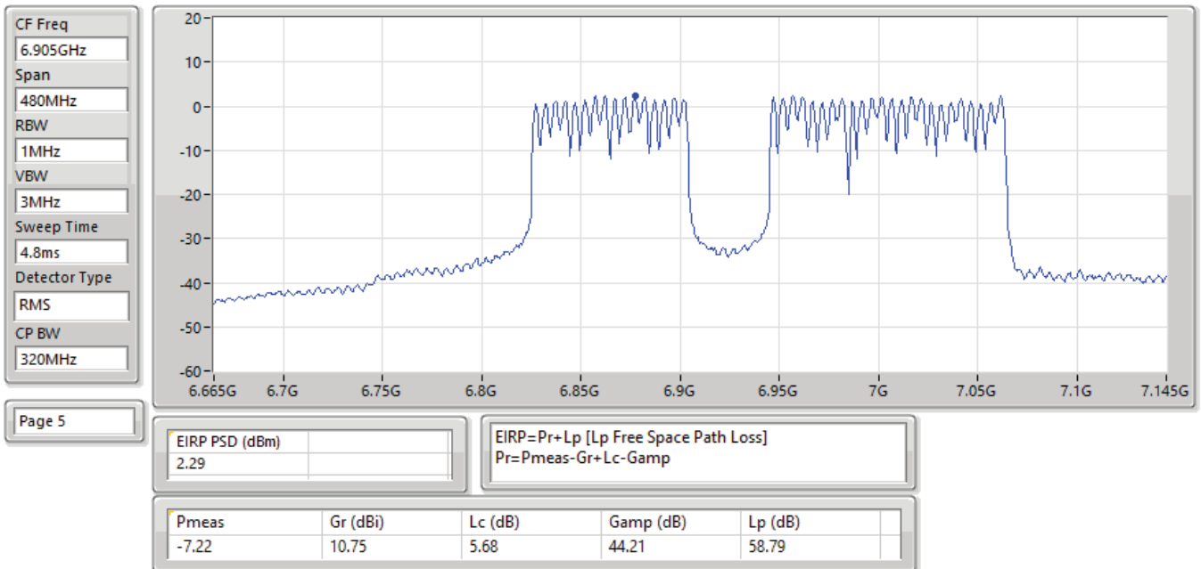
EIRP PSD;Band:6.7G;be320;BWch:320MHz;Nss:1,(M0),2xRU996+RU484 MRU 9;Nant:4;Ch:6905MHz;TX
