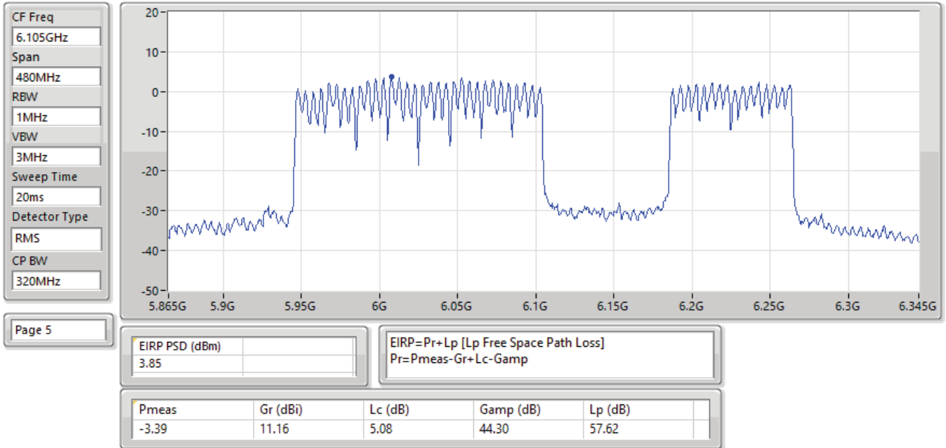
EIRP PSD;Band:6.2G;be320;BWch:320MHz;Nss:1,(M0),3xRU996 MRU 3;Nant:4;Ch:6105MHz;TX
