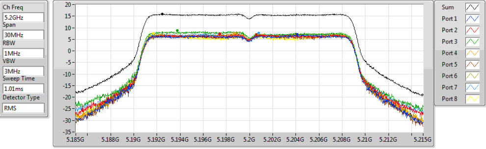
802.11ac VHT20-BF_Nss2,(MCS0)_8TX
