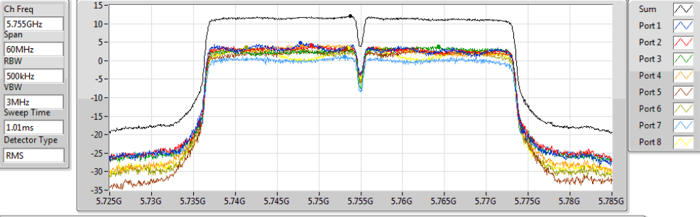
802.11ac VHT40-BF_Nss2,(MCS0)_8TX
