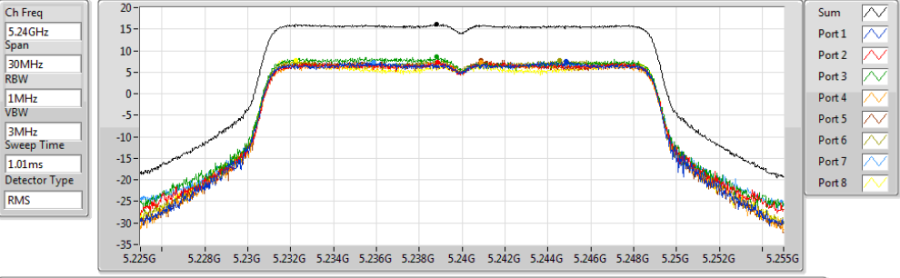
802.11ac VHT20-BF_Nss2,(MCS0)_8TX
