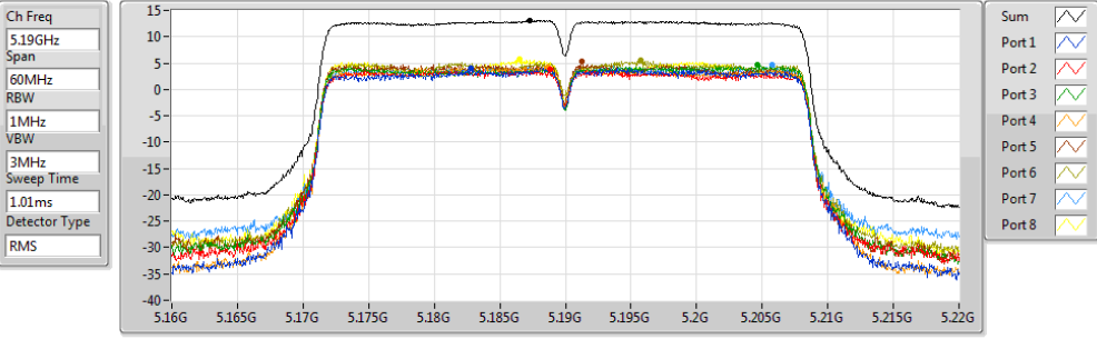
802.11ac VHT40-BF_Nss2,(MCS0)_8TX
