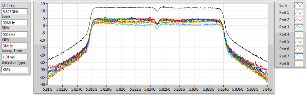
802.11ac VHT20-BF_Nss2,(MCS0)_8TX
