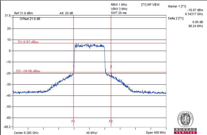
802.11ax (HE80) / Chain 2 : CH 87
