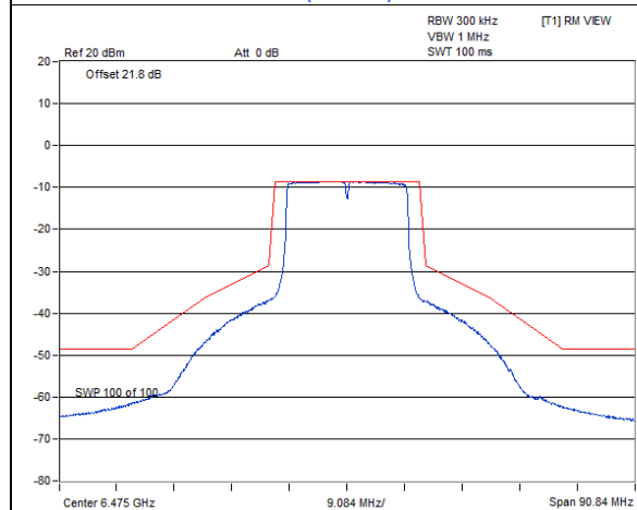
802.11ax (HE20) / Chain 0 : CH 105
