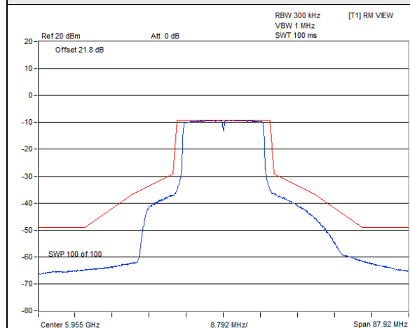
802.11ax (HE20) / Chain 0 : CH 1
