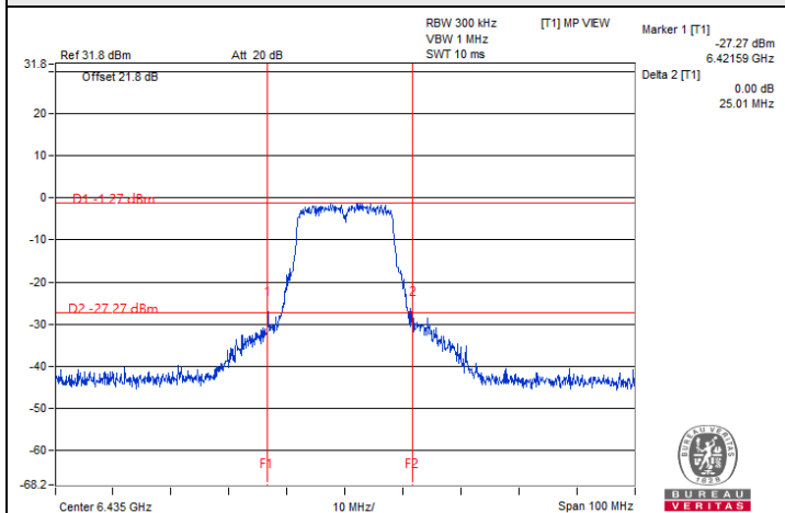
802.11a / Chain 2 : CH 97
