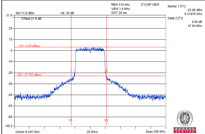
802.11ax (HE40) / Chain 3 : CH 99
