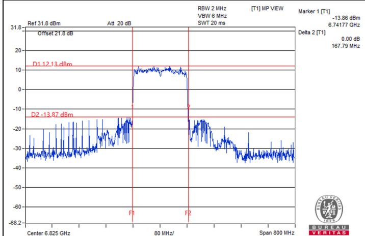
802.11ax (HE160) / Chain 3 : CH 175
