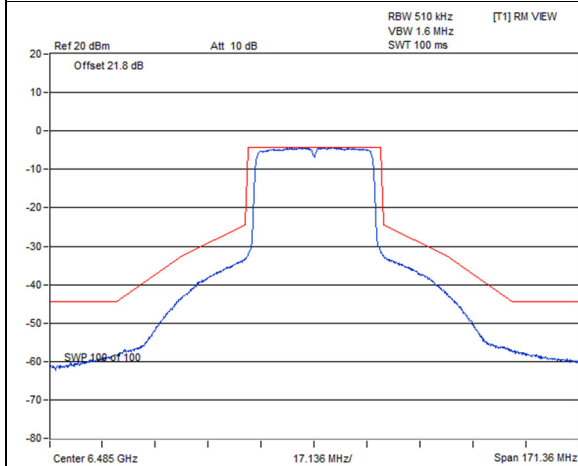
802.11ax (HE40) / Chain 2 : CH 107
