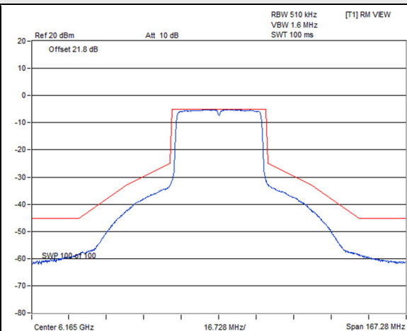
802.11ax (HE40) / Chain 2 : CH 43
