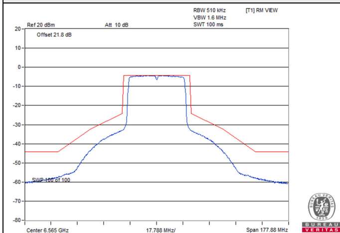
802.11ax (HE40) / Chain 3 : CH 123
