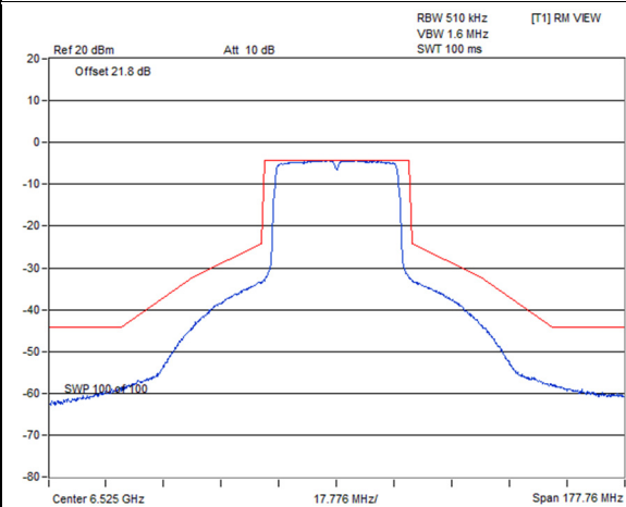
802.11ax (HE40) / Chain 2 : CH 115
