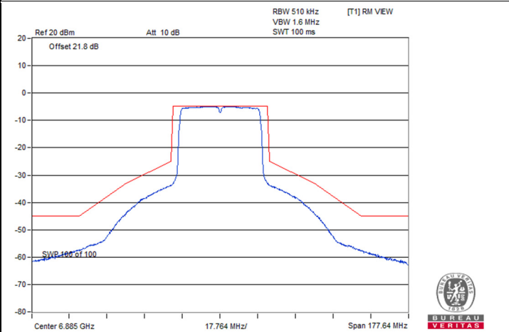
802.11ax (HE40) / Chain 2 : CH 187
