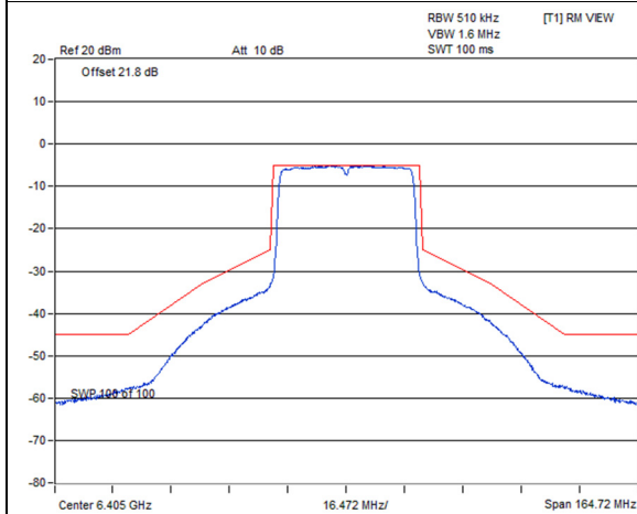
802.11ax (HE40) / Chain 2 : CH 91
