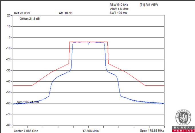
802.11ax (HE40) / Chain 3 : CH 227
