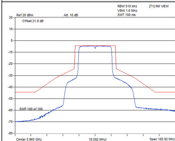
802.11ax (HE40) / Chain 2 : CH 3
