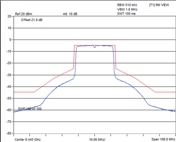
802.11ax (HE40) / Chain 2 : CH 99
