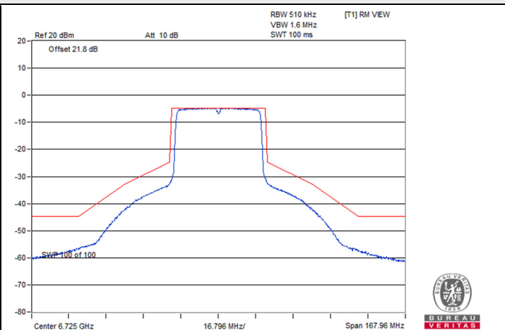
802.11ax (HE40) / Chain 2 : CH 155
