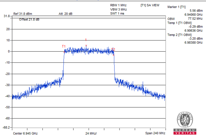
802.11ax (HE80) / Chain 0 : CH 199
