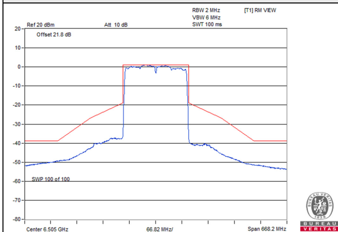
802.11ax (HE160) / Chain 3 : CH 111
