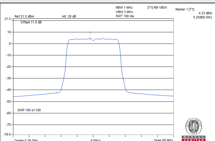
802.11ax (HE20) / Chain 3 : CH 52
