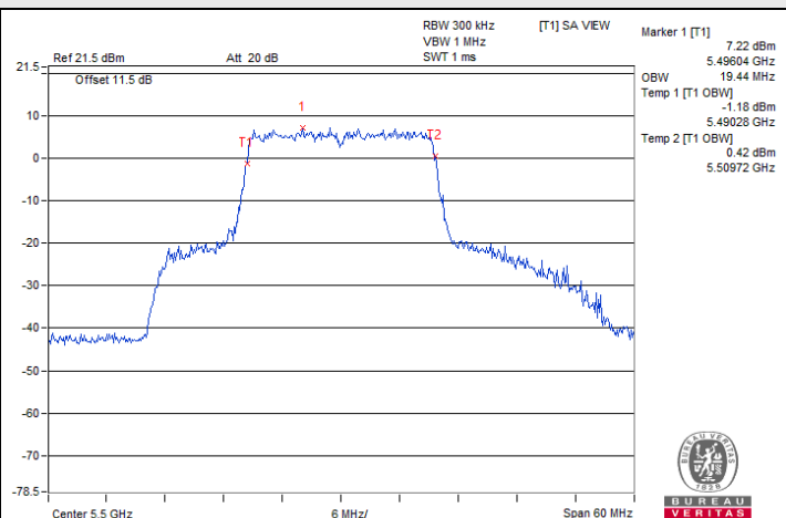
802.11ax (HE20) / Chain 2 : CH 100
