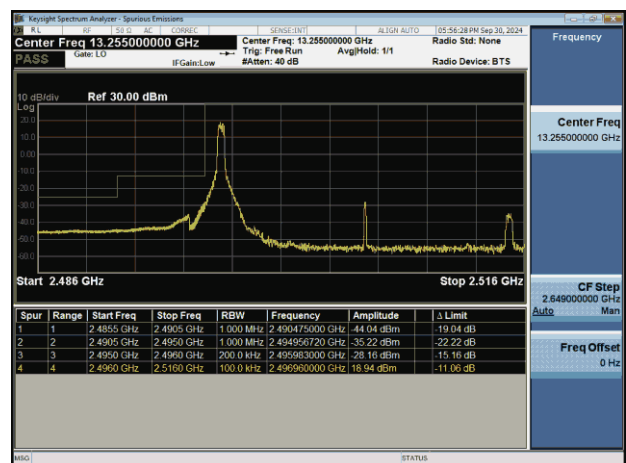
NTNV-n41-PC2-30-20-L-DFT-BPSK-Edge_1RB_Left-PASS
