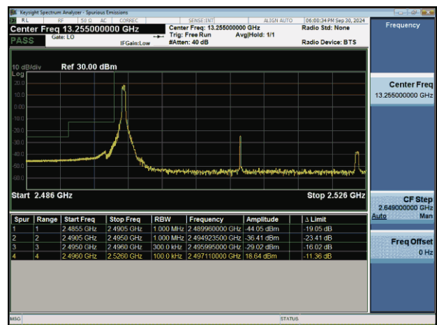
NTNV-n41-PC2-30-30-L-CP-QPSK-Edge_1RB_Left-PASS
