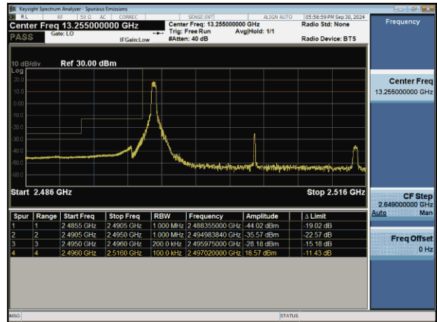
NTNV-n41-PC2-30-20-L-CP-QPSK-Edge_1RB_Left-PASS
