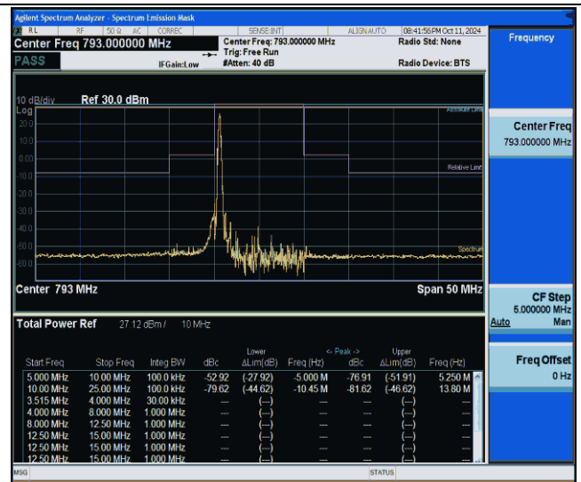
NTVN-Band14-10MHz-QPSK-23330-1RB#0--10.00--5.00-PASS
