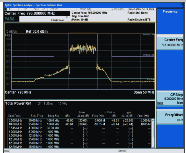
NTVN-Band14-10MHz-QPSK-23330-50RB#0--10.00--5.00-PASS
