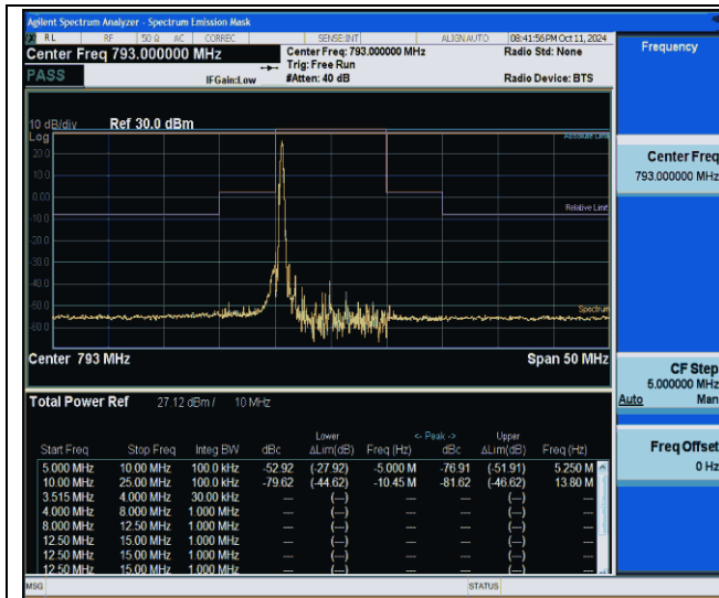
NTVN-Band14-10MHz-QPSK-23330-1RB#0--25.00--10.00-PASS
