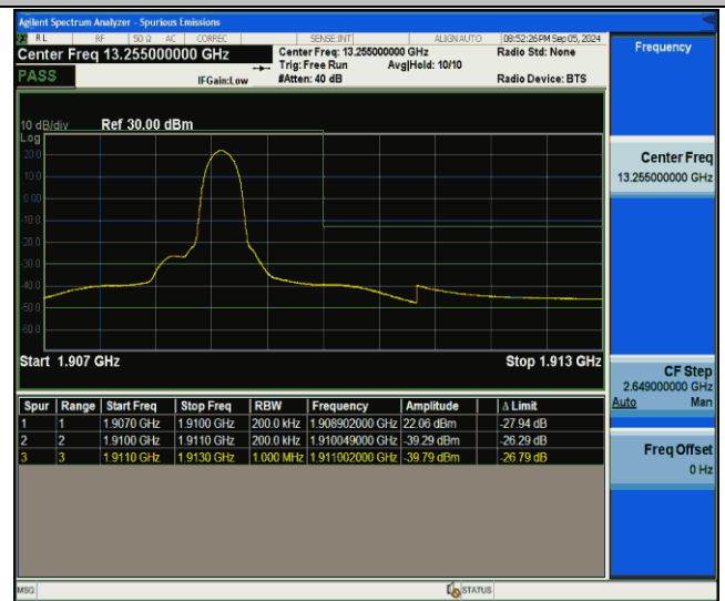
Band2-20MHz-QPSK-19100-1RB#99-PASS
