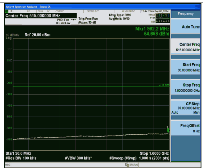
Band25-20MHz-QPSK-26365-1RB#0-30~1000-PASS
