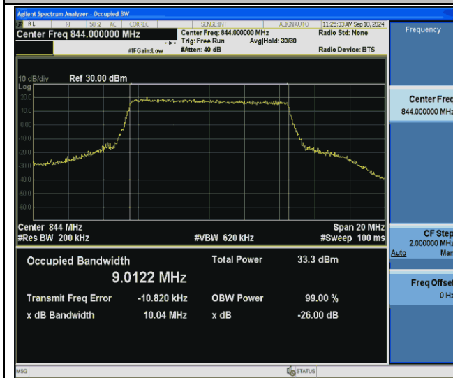
Band26(824-849)-10MHz-QPSK-26990-50RB#0-PASS
