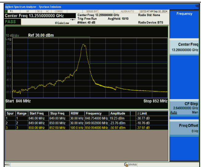
Band26(824-849)-3MHz-QPSK-27025-1RB#14-PASS
