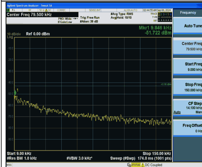
Band66-20MHz-QPSK-132572-1RB#0-0.009~0.15-PASS
