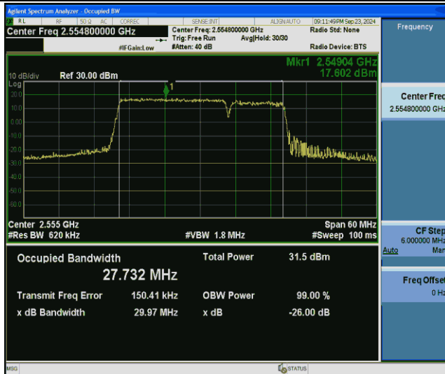
7-7-20MHz-10MHz-QPSK-QPSK-21251-21395-100RB#0- 50RB#0-PASS
