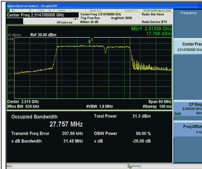
7-7-20MHz-10MHz-QPSK-QPSK-20850-20994-100RB#0- 50RB#0-PASS
