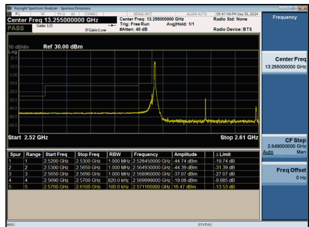
NTNV-n38-PC3-30-40-L-CP-QPSK-Edge_1RB_Left-PASS
