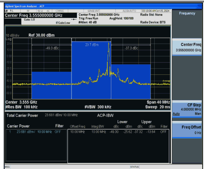
Band48-10MHz-QPSK-55290-1RB#49-PASS
