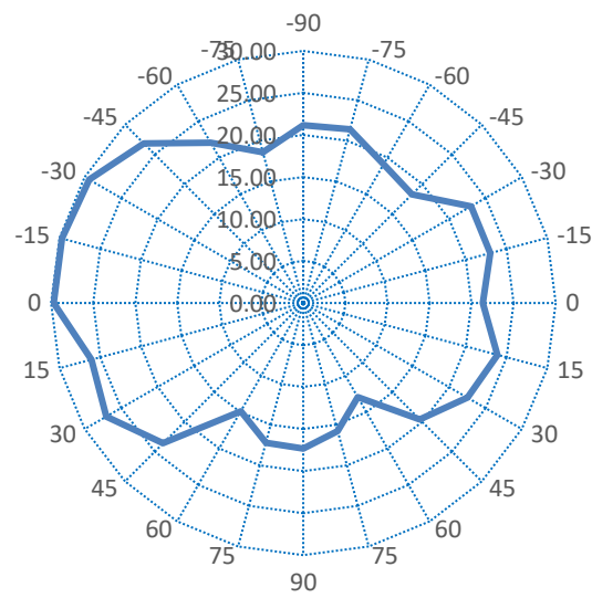
5G Ch100
