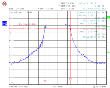
903MHz
