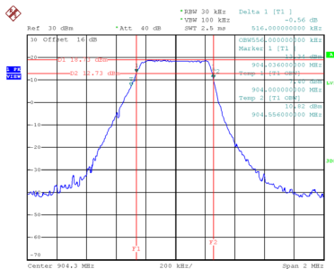
904.3MHz
