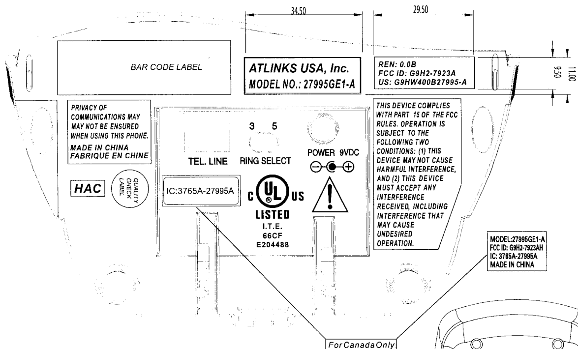
27995GE1-A LABEL DRAWING DATE : 05 JAN, 2005
