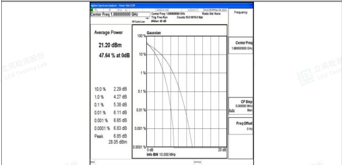
Band2-10MHz-QPSK-18900-50RB#0-PASS
