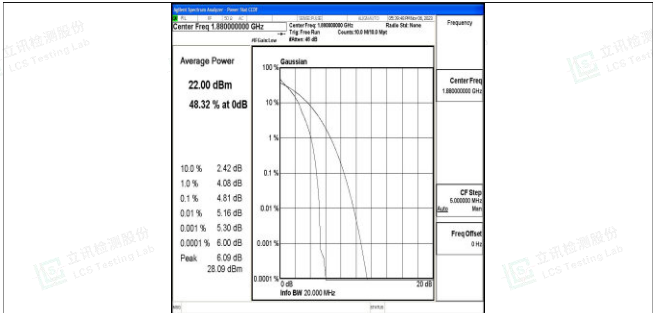
Band2-20MHz-QPSK-18900-1RB#0-PASS
