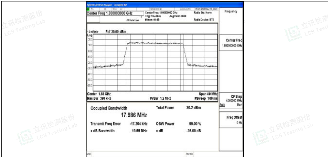
Band2-20MHz-QPSK-18900-100RB#0-PASS
