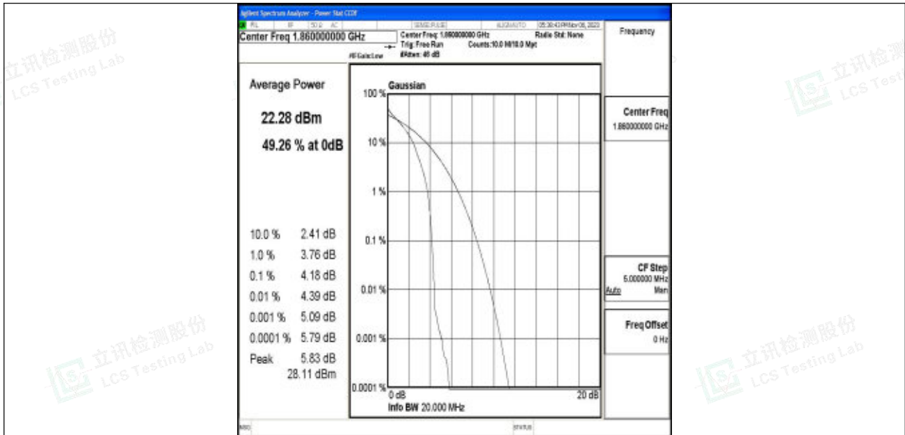
Band2-20MHz-64QAM-18700-1RB#0-PASS
