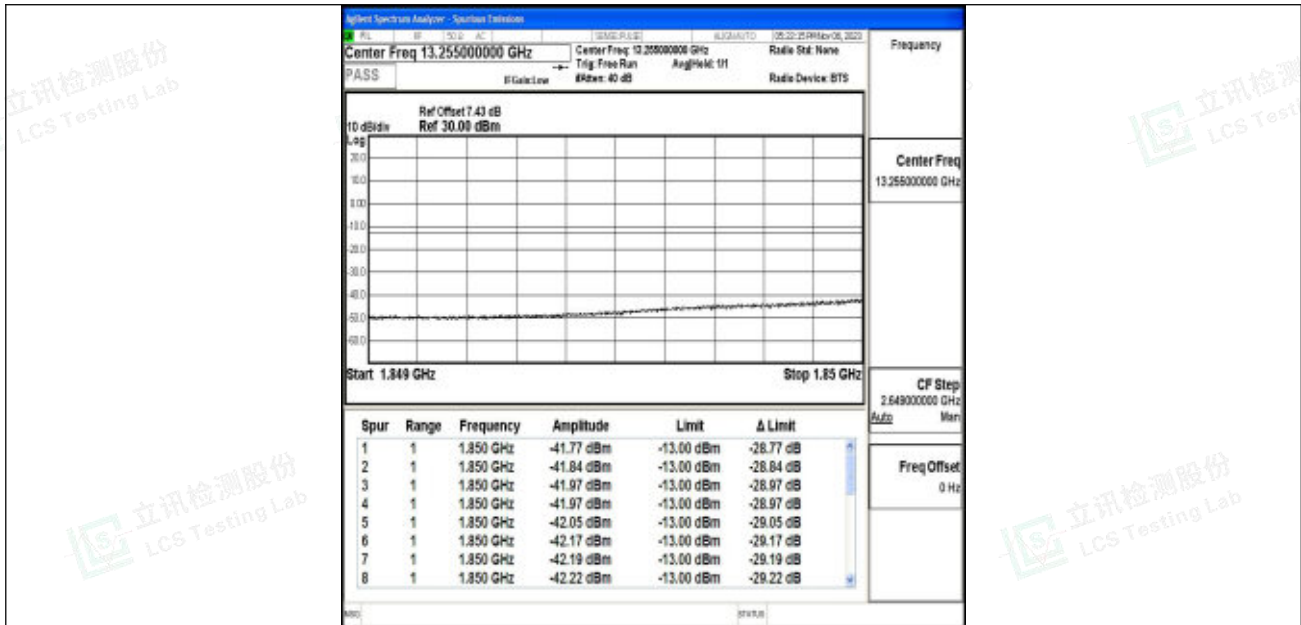
Band2_20MHz_QPSK_18700_1RB#0
