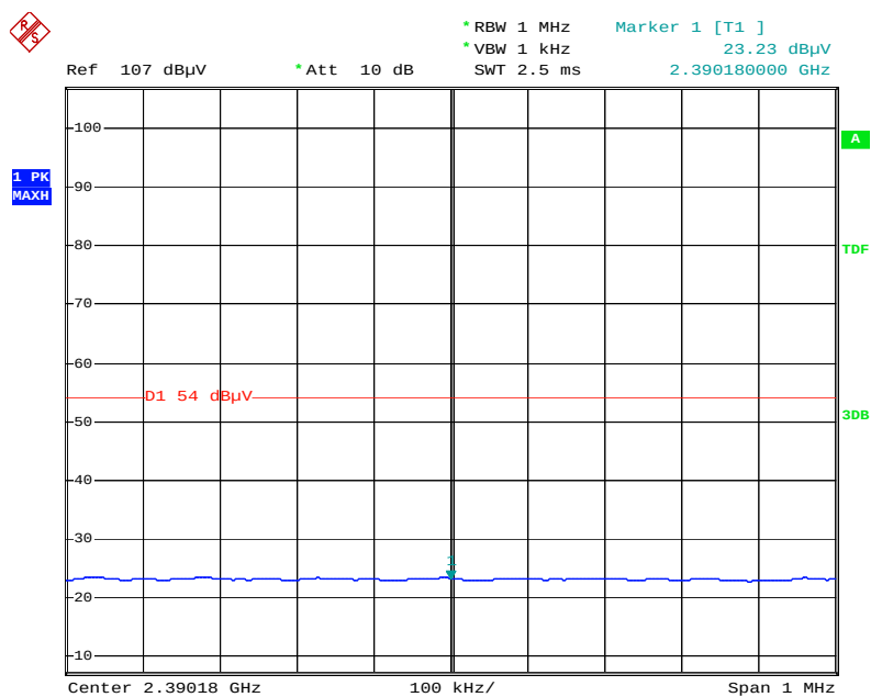
GFSK-hopping-Av-Left
