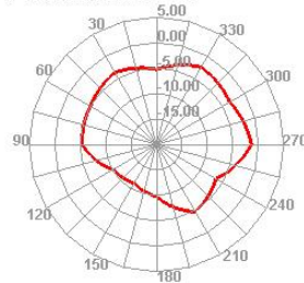
5490.000MHz E2
