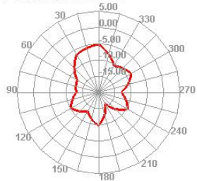
5490.000MHz E1
