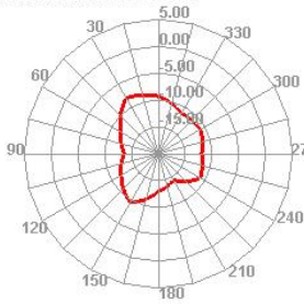
5850.000MHz E1
