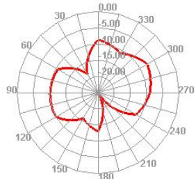
5150.000MHz E1
