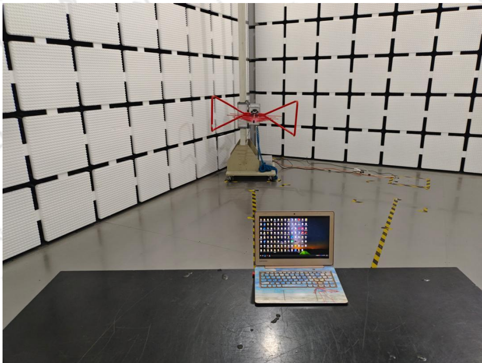
30MHz-1000MHz
