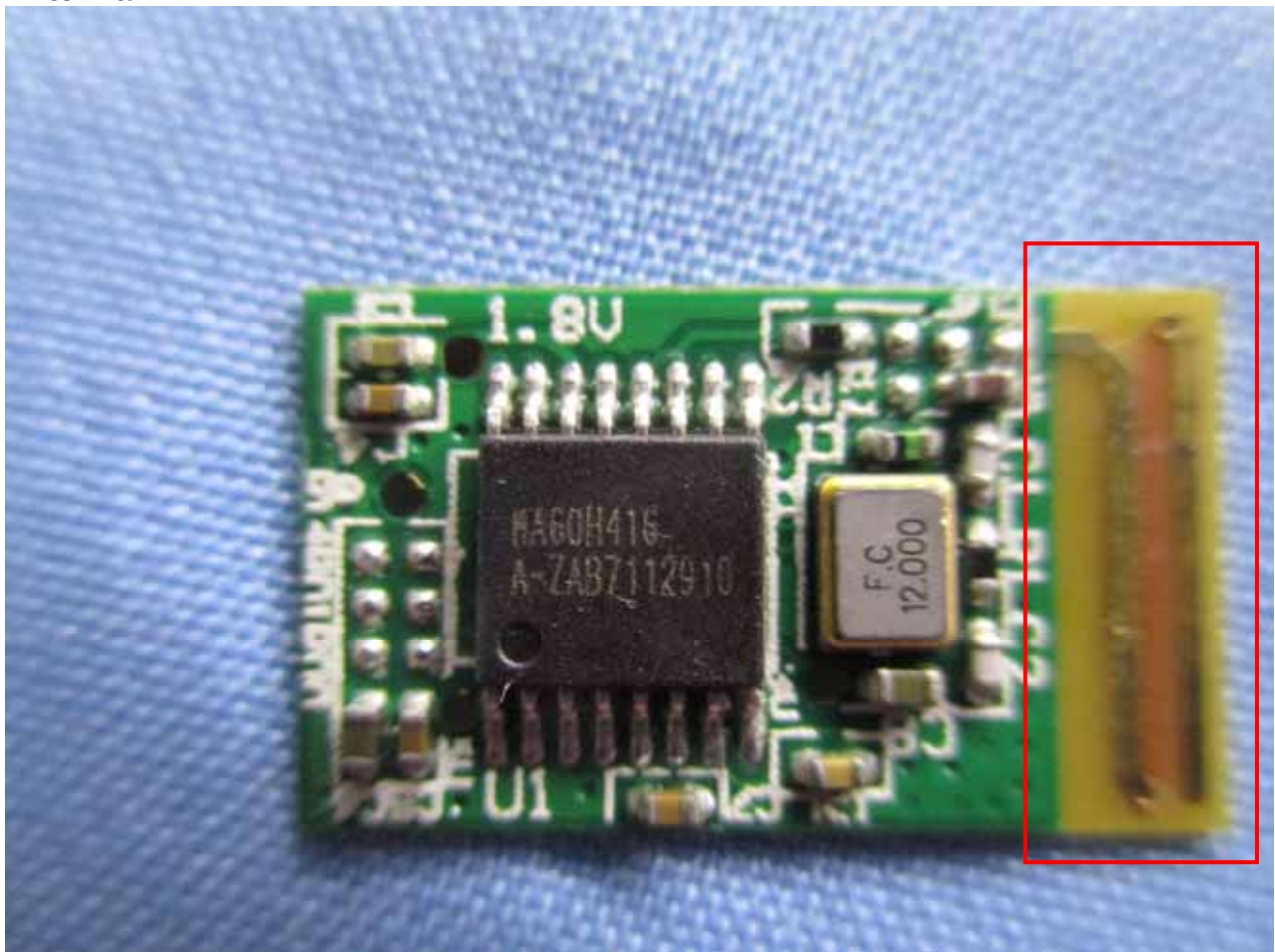
Antenna
