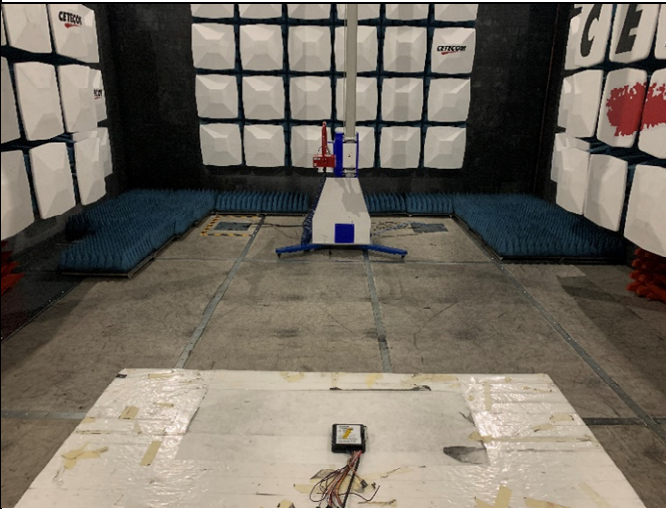
9kHz – 30MHz
