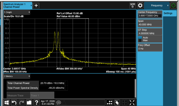
QPSK CH 56690 (3695 MHz)
