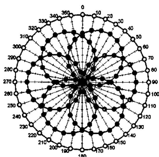
f = 900 \text{ MHz} , TEM cell if110
