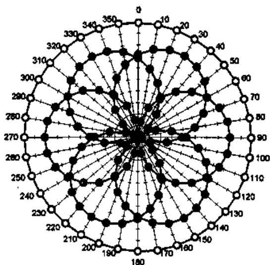
f = 300 \text{ MHz} , TEM cell if110
