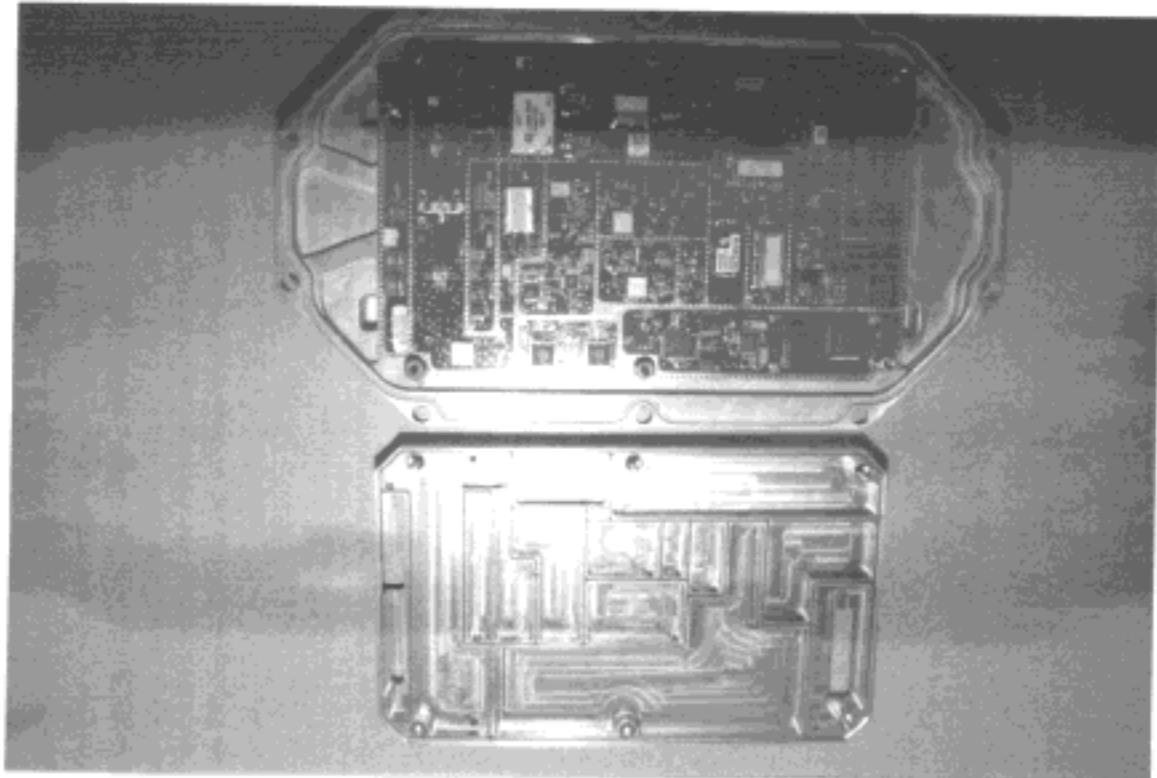
DIGITAL PCA & 8.4 GHZ COVER REMOVED, 8.4 GHZ RF PCA
