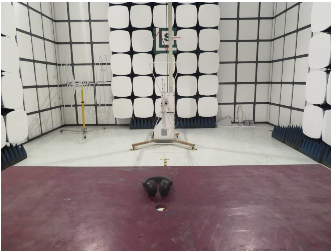
Above 1G
