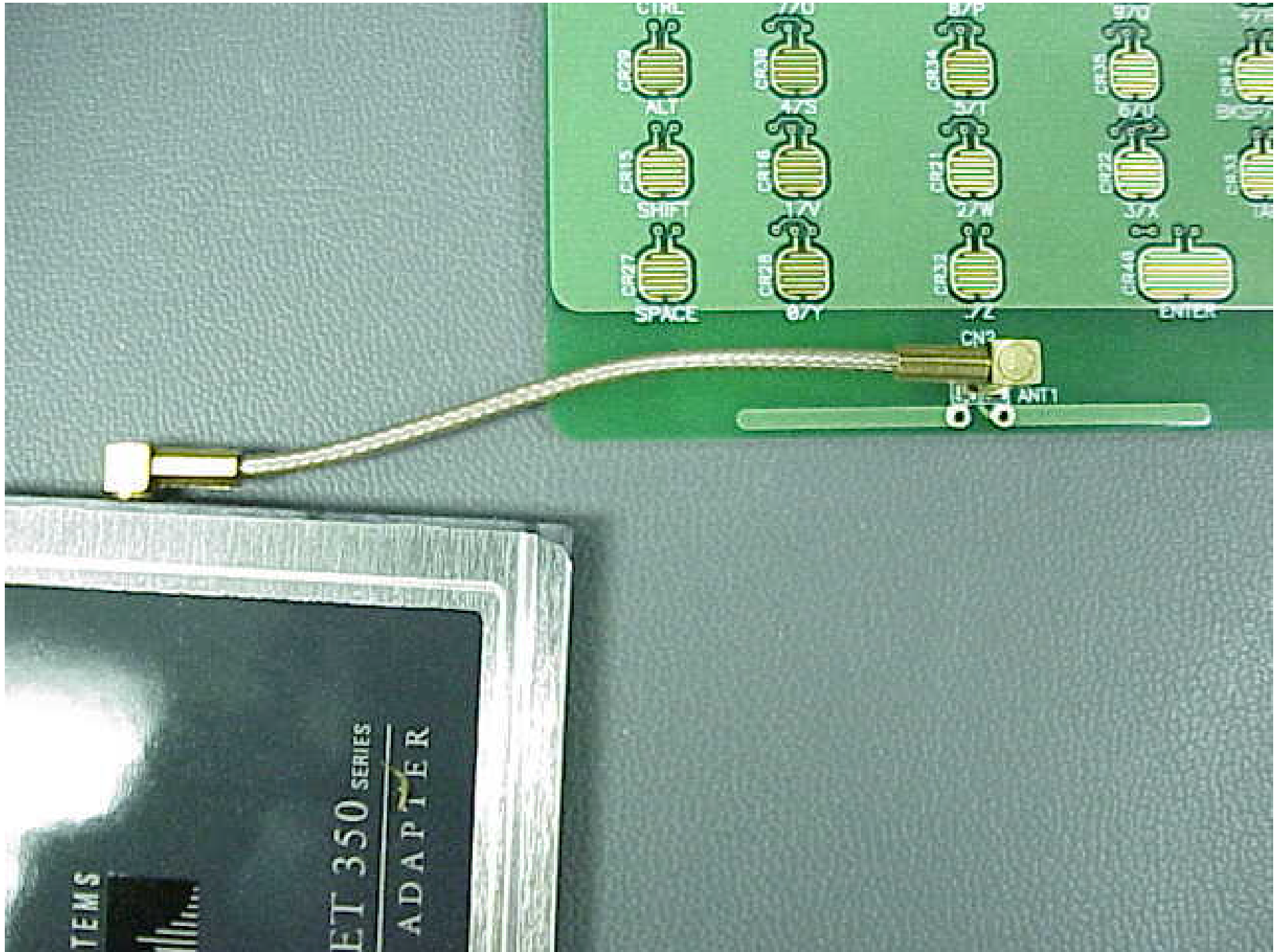
Antenna
