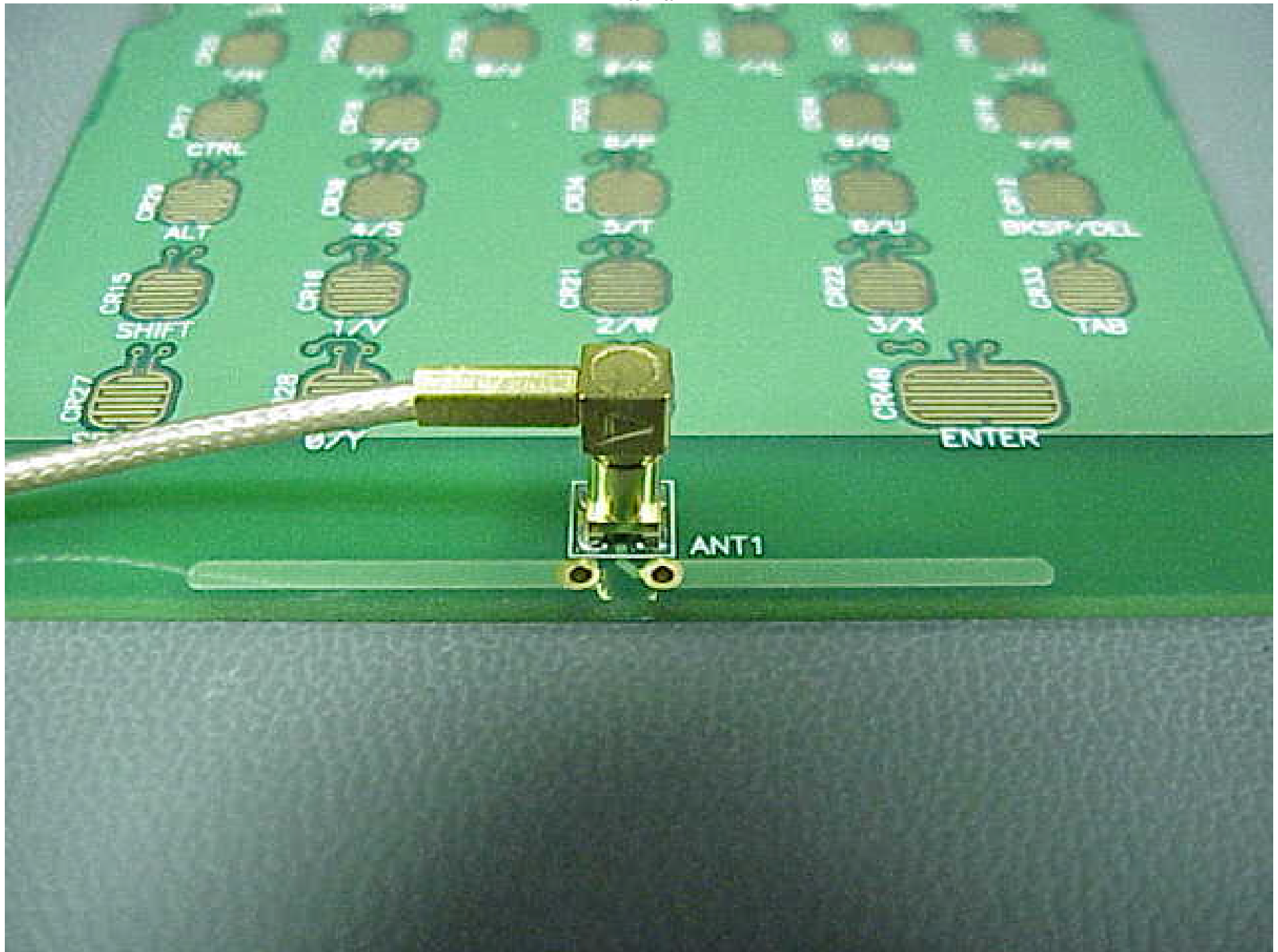
Antenna
