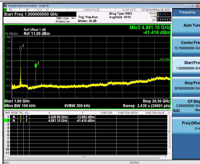
2.4G_Ant1_2440_1000~26500
