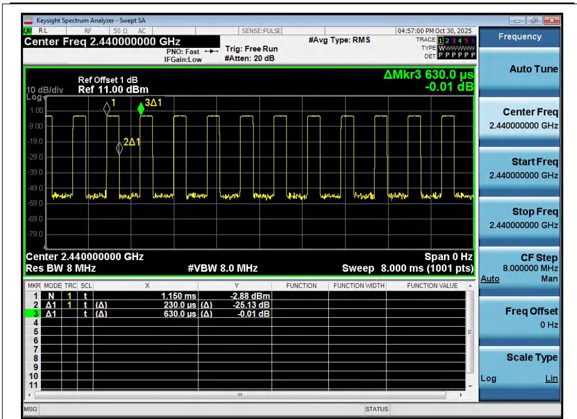
NTNV-BLE_2M-Ant1-2440
