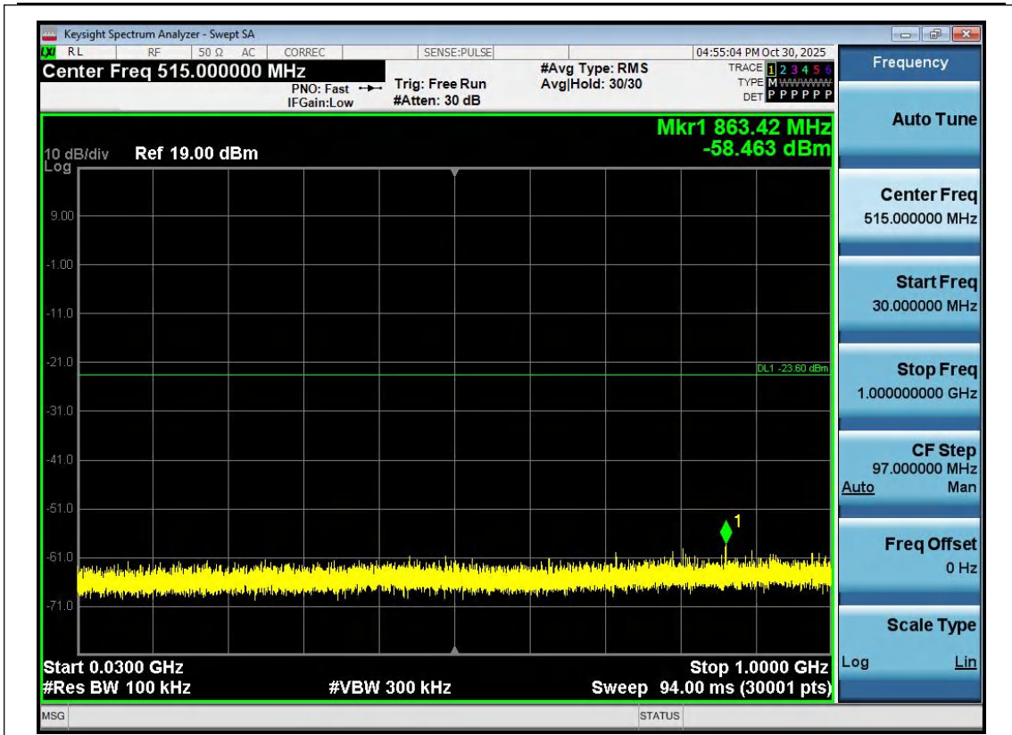
BLE_2M-Ant1-2402-30~1000-PASS
