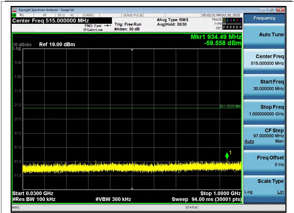
BLE_2M-Ant1-2480-30~1000-PASS
