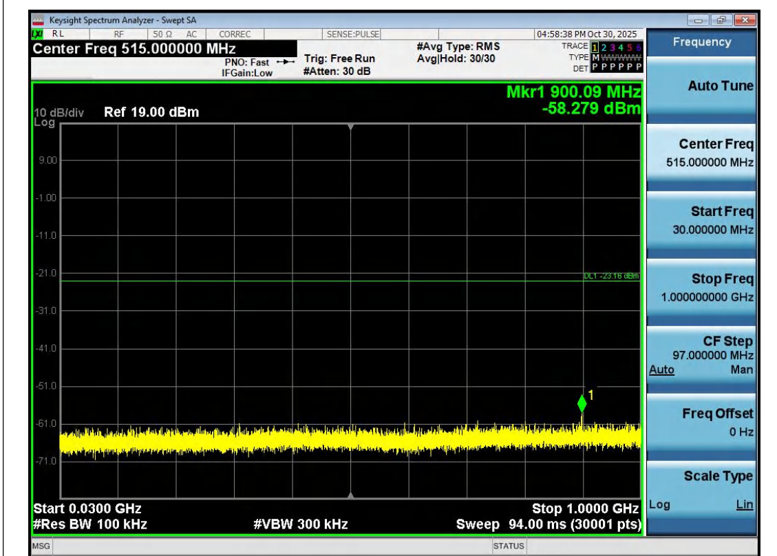
BLE_2M-Ant1-2440-30~1000-PASS
