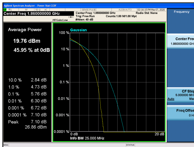
Band2-20MHz-16QAM-18700-100RB#0
