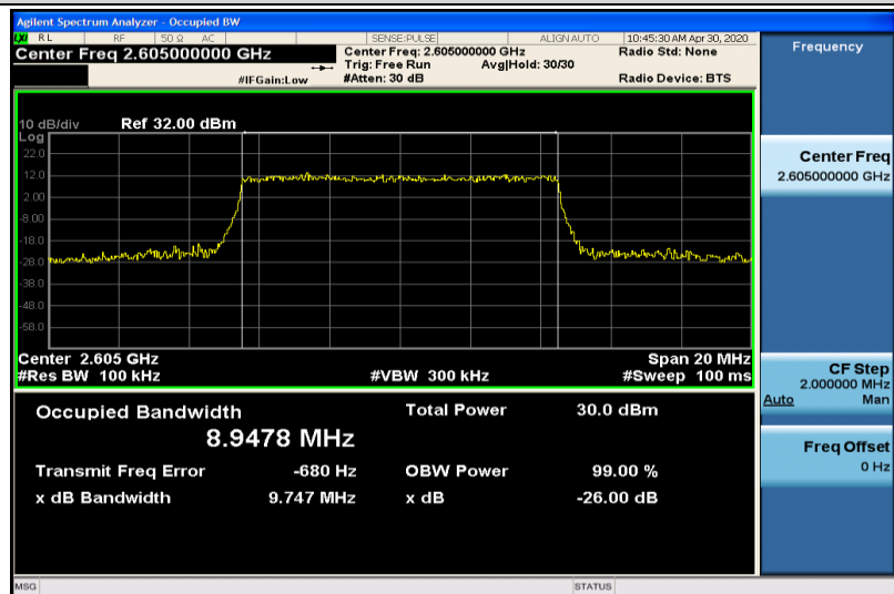
Band41-10MHz-QPSK-40740-50RB#0-8.9478
