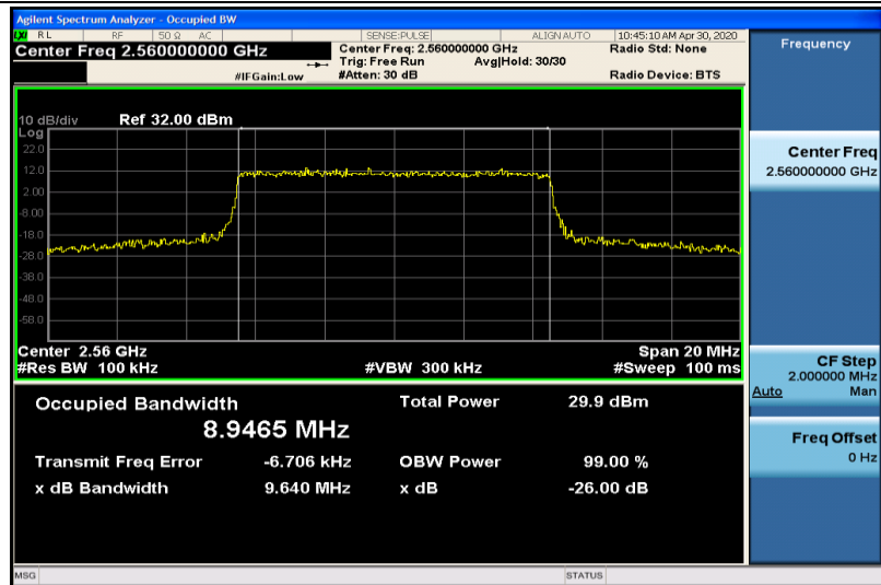
Band41-10MHz-QPSK-40290-50RB#0-8.9465
