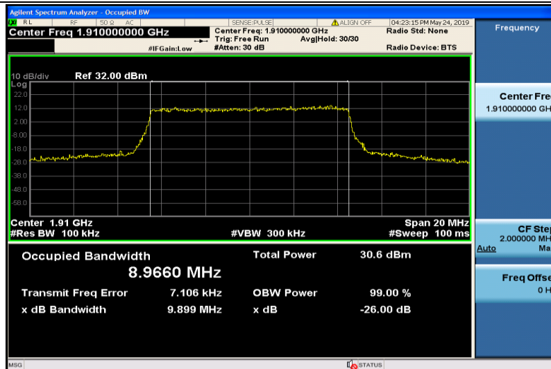
Band25-10MHz-QPSK-26640-50RB#0-8.9660
