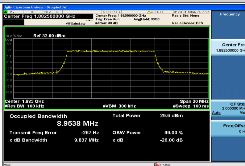
Band25-10MHz-16QAM-26365-50RB#0-8.9538
