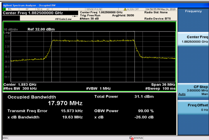
Band25-20MHz-QPSK-26365-100RB#0-17.970
