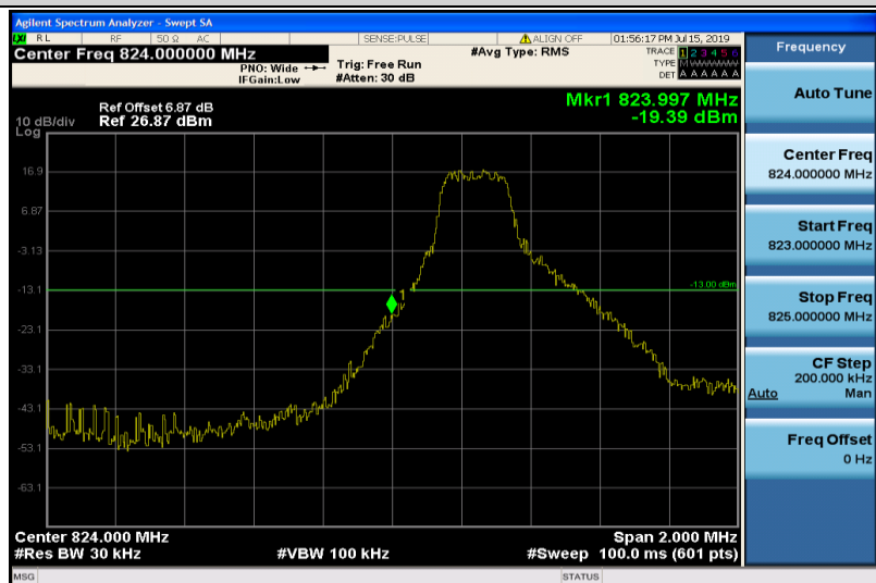
Band5-3MHz-QPSK-20415-1RB#0
