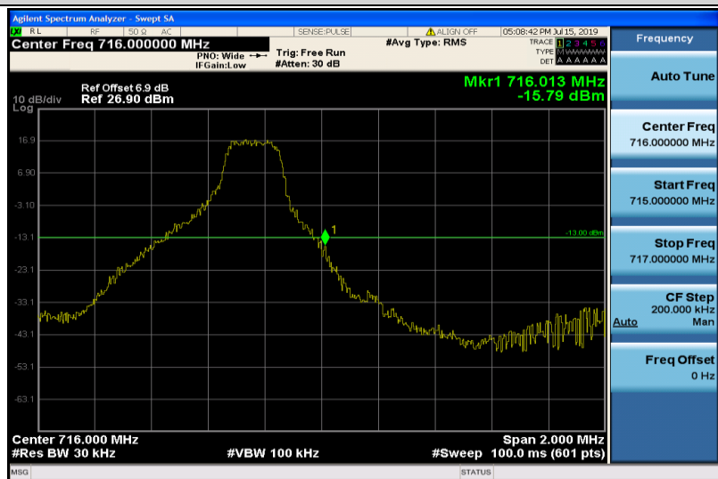
Band12-3MHz-QPSK-23165-1RB#14
