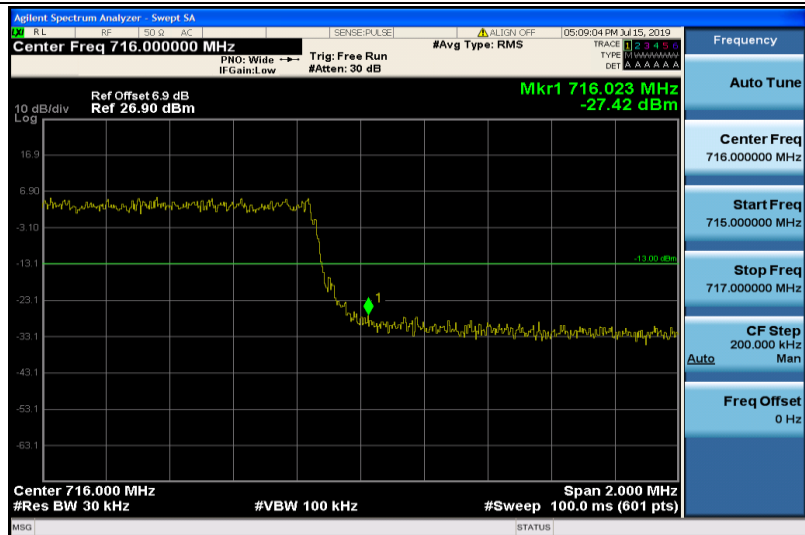
Band12-3MHz-QPSK-23165-15RB#0
