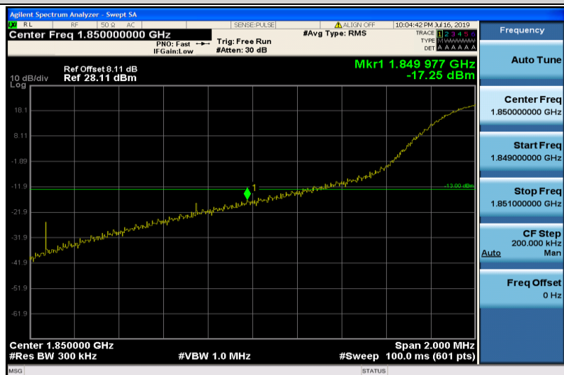
Band25-20MHz-QPSK-26140-1RB#0
