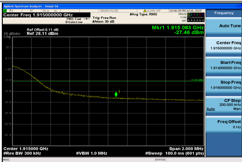
Band25-20MHz-QPSK-26590-100RB#0
