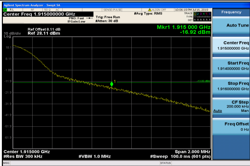
Band25-20MHz-QPSK-26590-1RB#99
