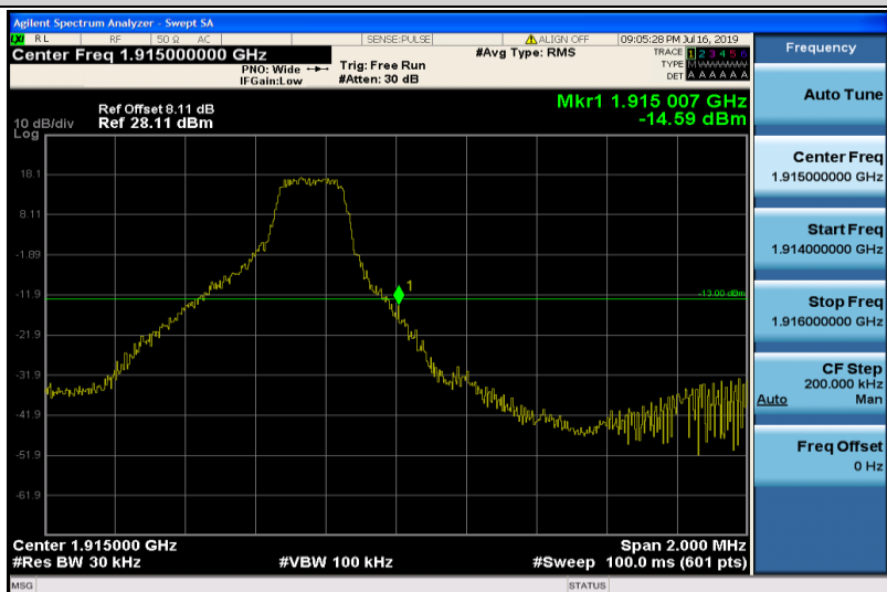
Band25-3MHz-QPSK-26675-1RB#14
