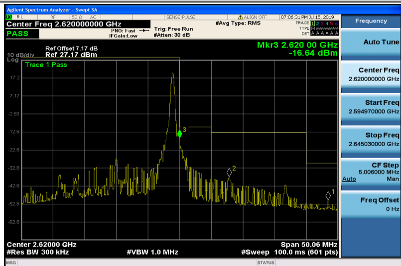
Band38-20MHz-QPSK-38150-1RB#99
