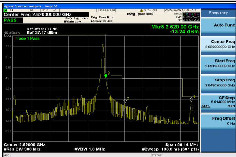
Band38-15MHz-QPSK-38175-1RB#74
