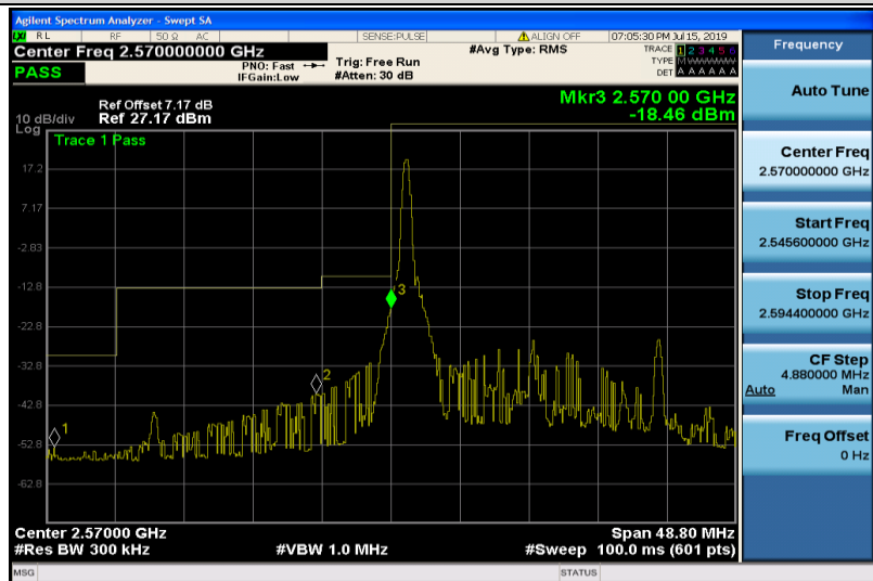
Band38-20MHz-QPSK-37850-1RB#0
