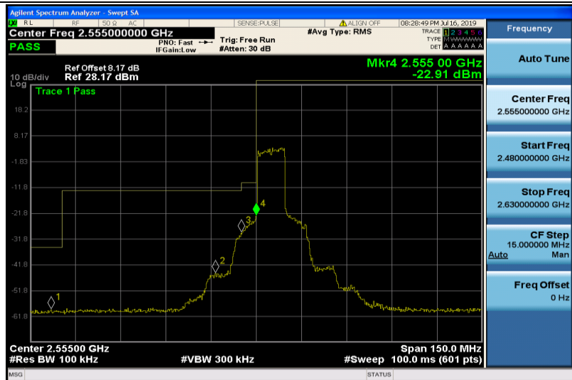
Band41-10MHz-QPSK-40290-1RB#0
