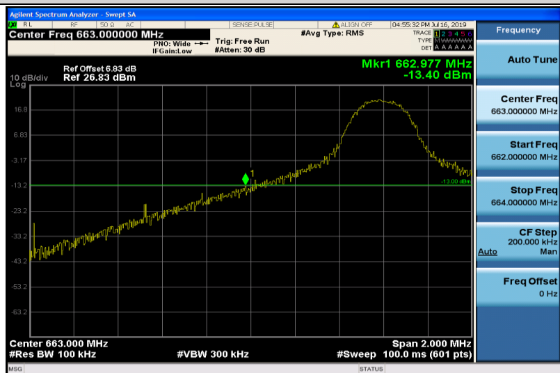
Band71-10MHz-QPSK-133172-1RB#0
